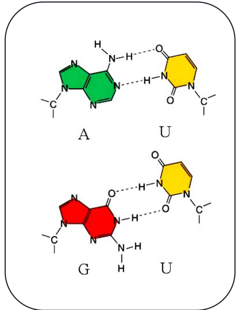
Uracil
